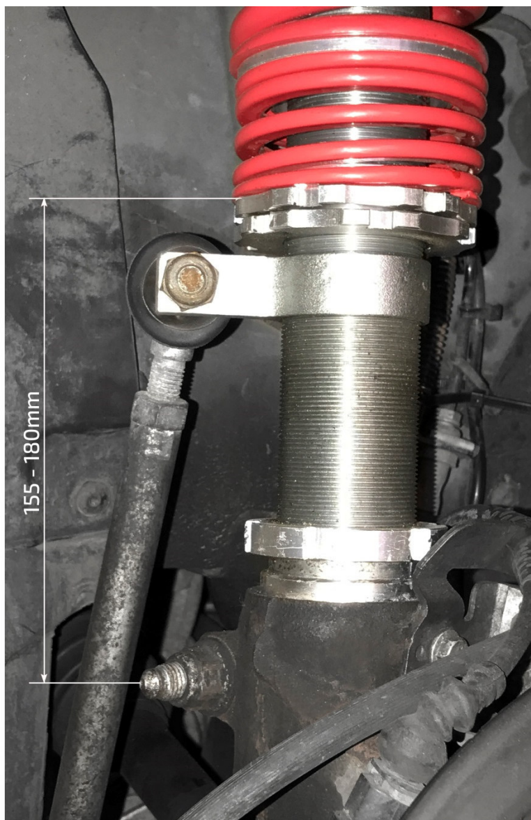
Fahrwerk Achse 1
