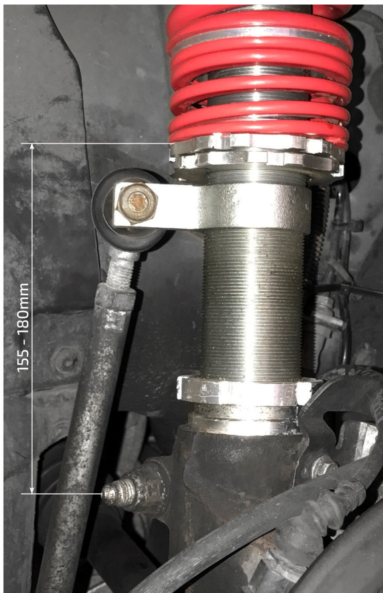
Fahrwerk Achse 1
