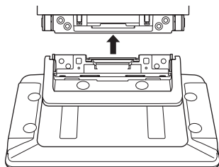
Schrauben (M5×8) (mitgeliefert)
